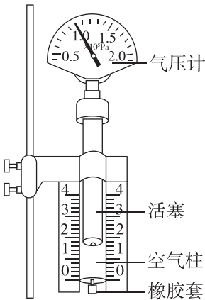
实验装置示意图
